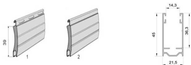
Lame perforée Lame non perforée
